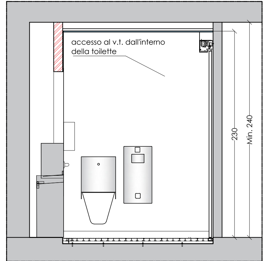
SEZIONE A:A'
